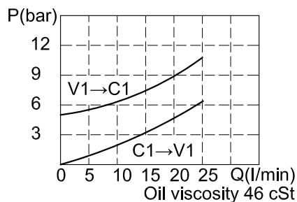
RATING DIAGRAM 流速表
