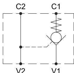
HYDRAULIC DIAGRAM 油路符號
