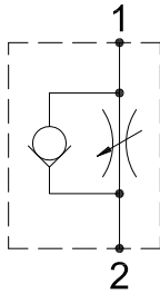
HYDRAULIC DIAGRAM 油路符號
