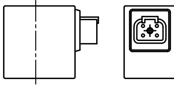
D16-05-12-28 Connection=Deutsch connection 德规电磁线圈
