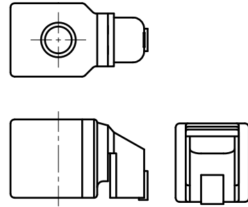
D13-08-24-26 Connection=Deutsch connection 德规电磁线圈
