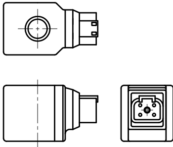
D13-05-24-26 Connection=Deutsch connection 德规电磁线圈
