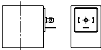
D16-01-12-28 Connection=A EN 175301-803 ISO 4400(DIN.43650) 电磁线圈
