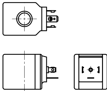
D13-01-12-26 Connection=A EN 175301-803 ISO 4400(DIN.43650) 电磁线圈
